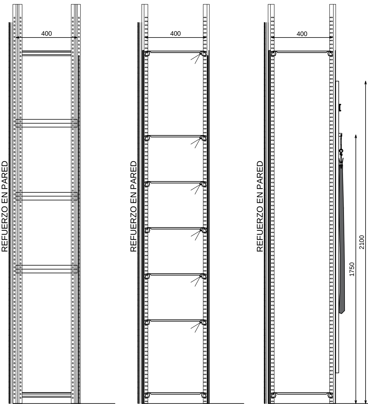
ALZADO LATERAL
