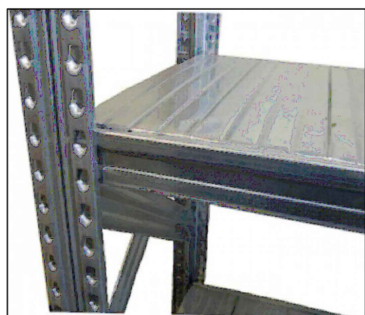
*REFERENCIA MONTANTES
