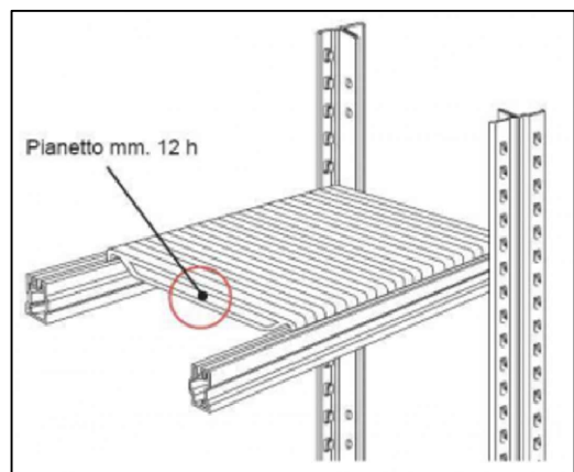
*REFERENCIA MONTANTES
