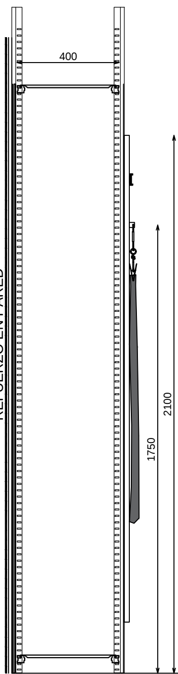
SECCIÓN CHAPA FRONTAL
