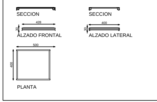
DETALLE MODULO 80
