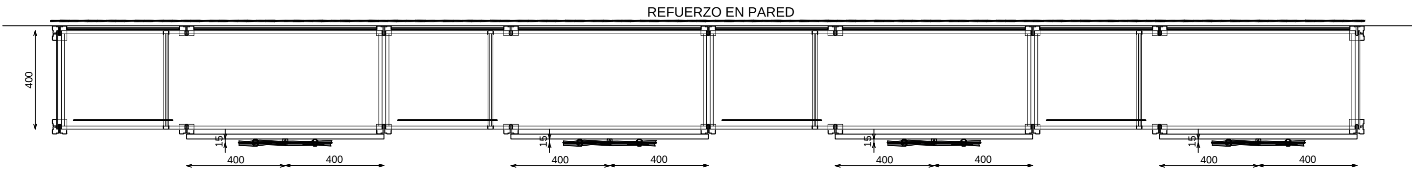
PLANTA SECCIONADA (PERCHA)
