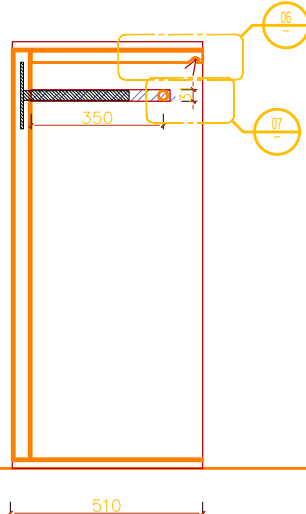
4:1:10 剖面图 SECTION
