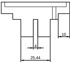
SECCIÓN PERFIL
