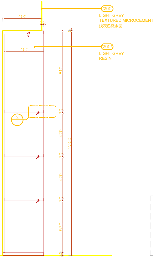
3 剖面图 1:10 SECTION
