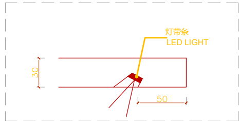
4 节点 1:2 DETAIL
