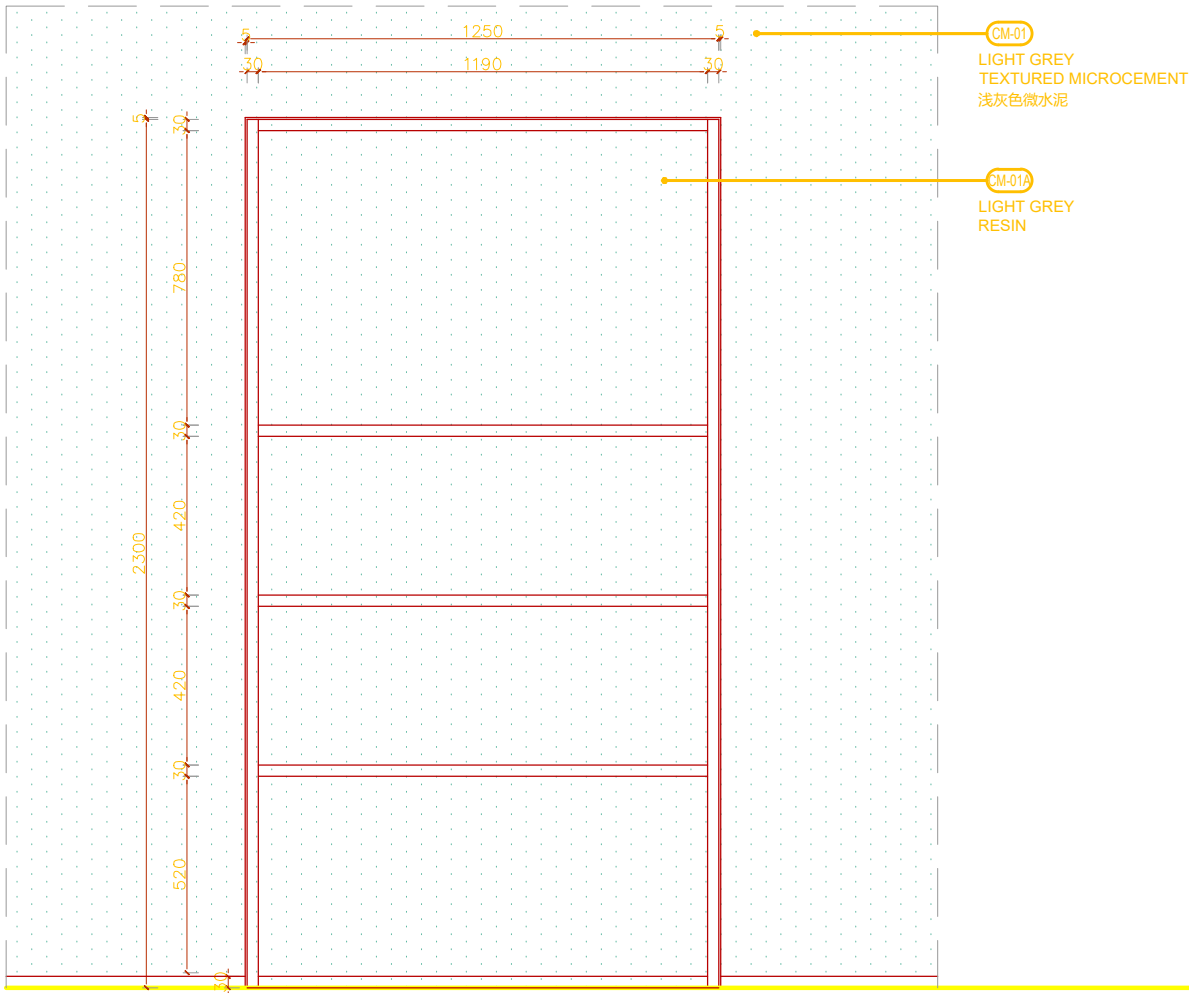
2 正立面 1:10 FRONT ELEVATION
