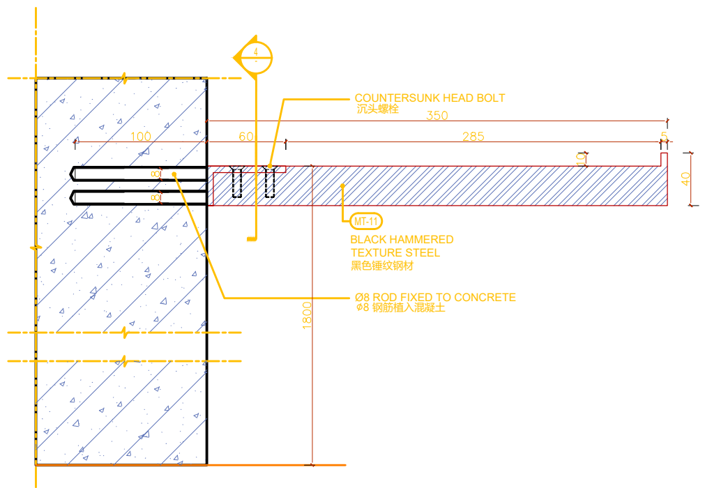
2 支撑杆件放大正立面 1:2 BAR HOLDER ENLARGE FRONT ELEVATION
