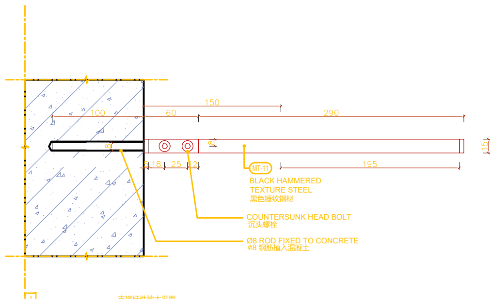
1 支撑杆件放大平面 1:2 BAR HOLDER ENLARGE PLAN
