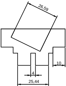
SECCIÓN PERFIL
