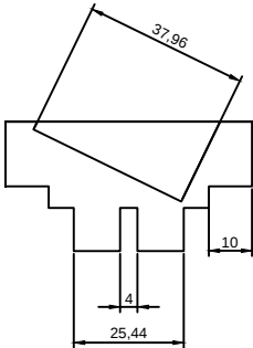
SECCIÓN PERFIL
