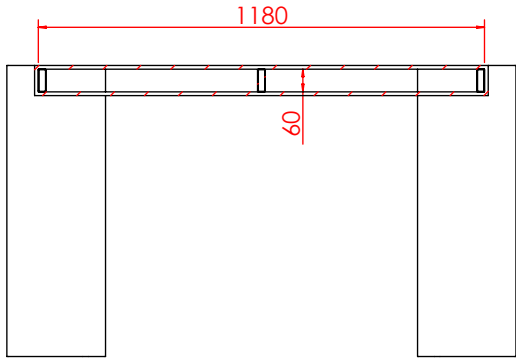
剖面 AH-AH
