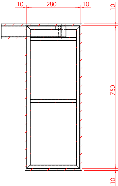
剖面 AI-AI 比例 1 : 10
