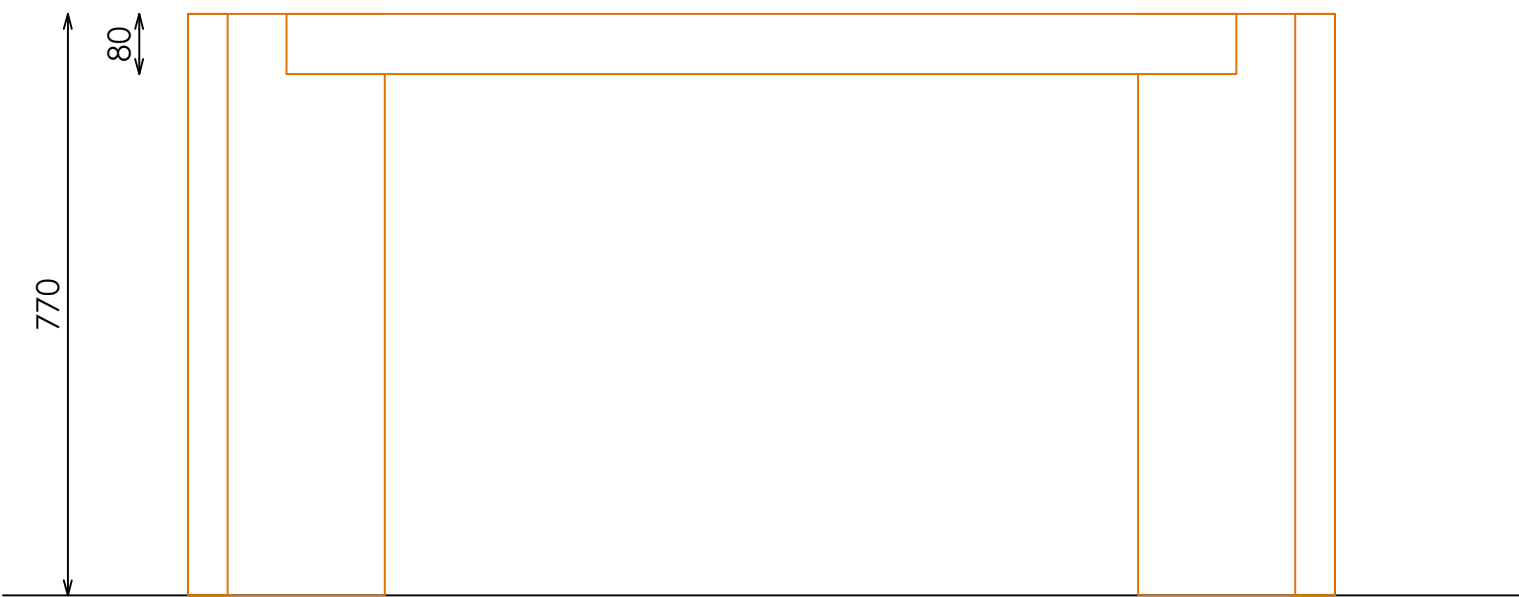
ALZADO FRONTAL
