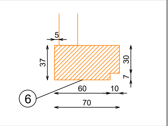
DETALLE FRONTALES EXTRAIBLES (TUBO MACIZO)
