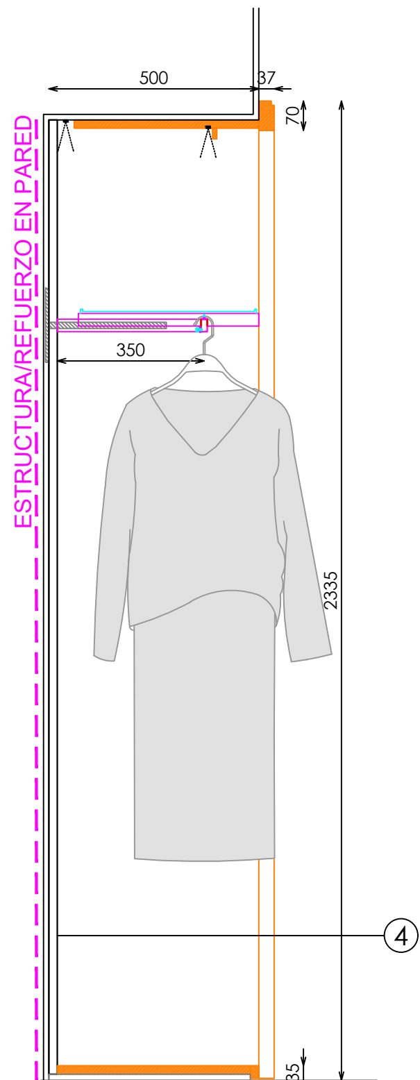
SECCIÓN BARRA ALTA
