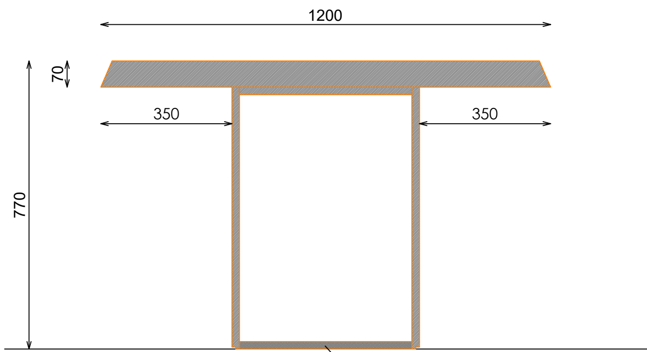
SECCION LATERAL
