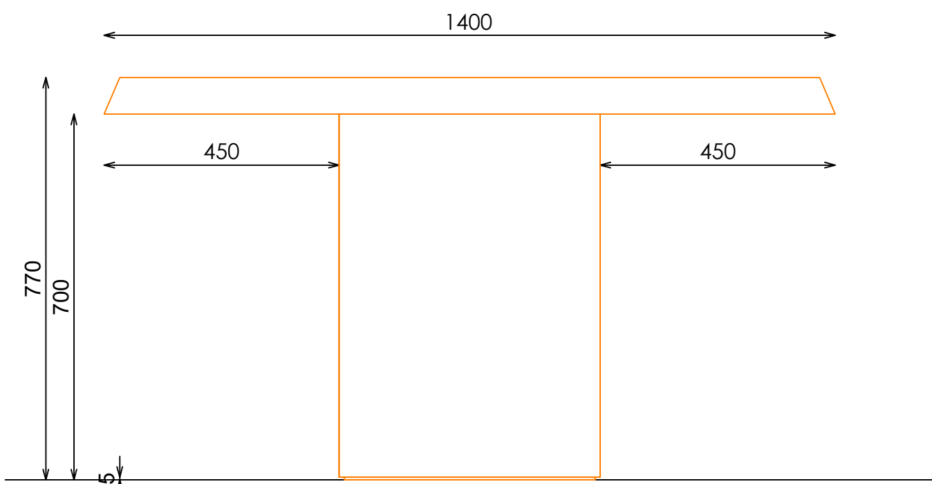
ALZADO FRONTAL
