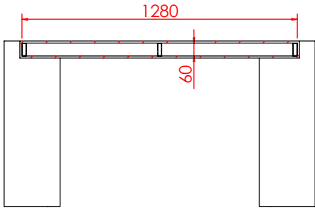
剖面 AH-AH
