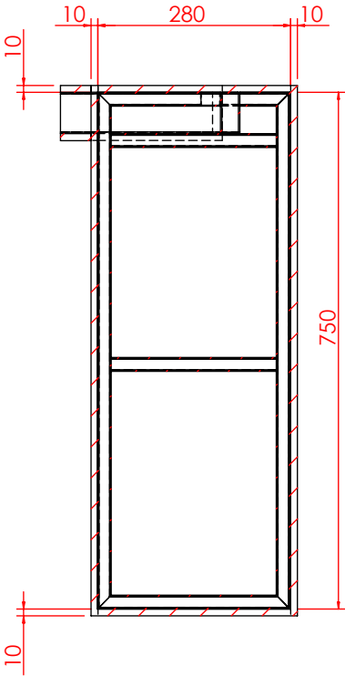
剖面 AI-AI 比例 1 : 10
