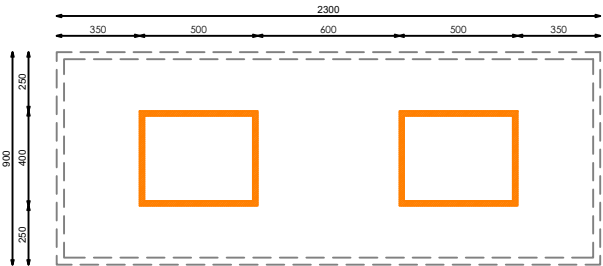
PLANTA SECCIONADA
