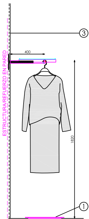
SECCIÓN BARRA
