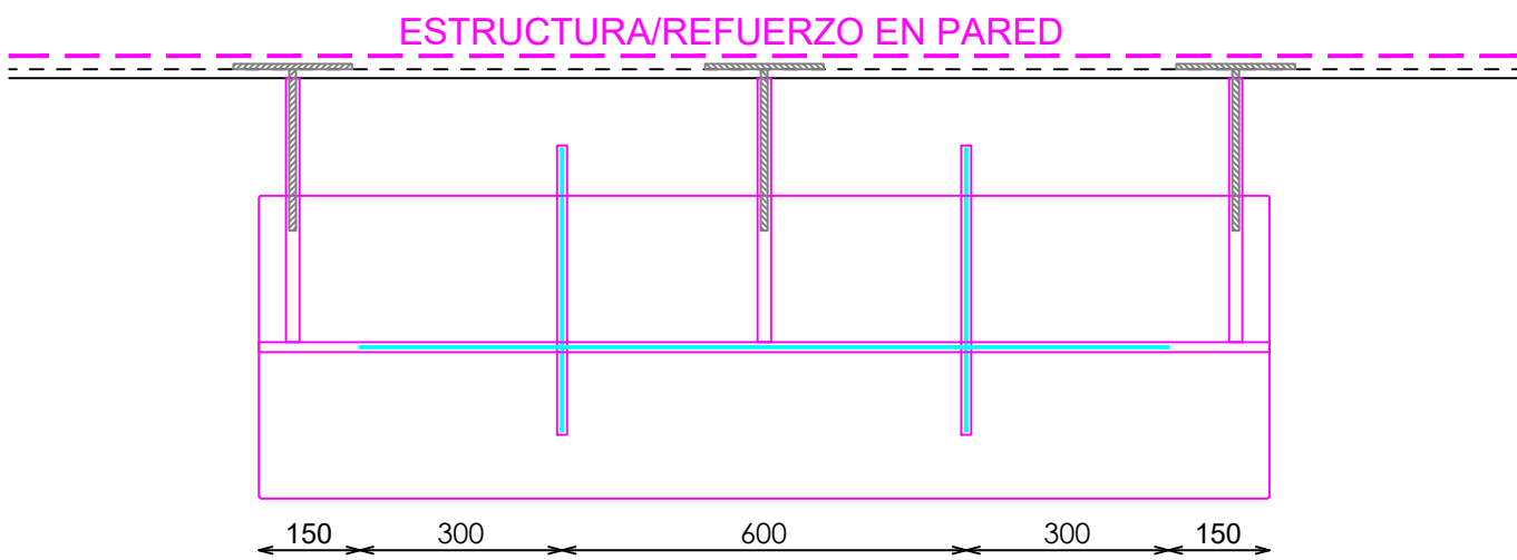
PLANTA
