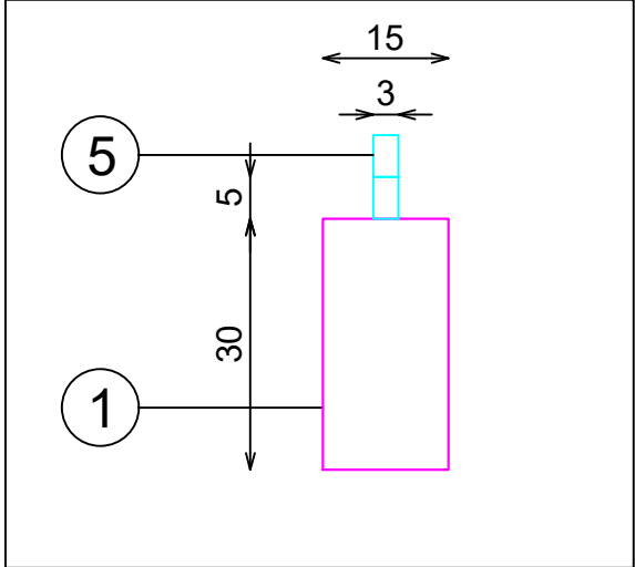
DETALLE BARRA
