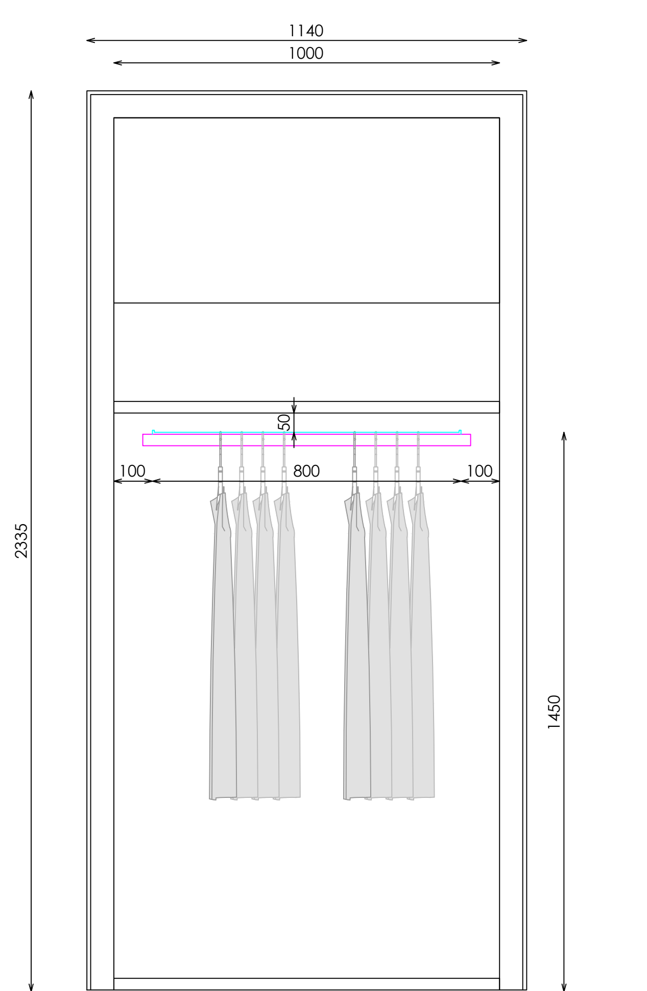
ALZADO
