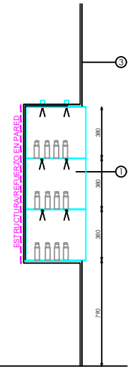
SECCIÓN
