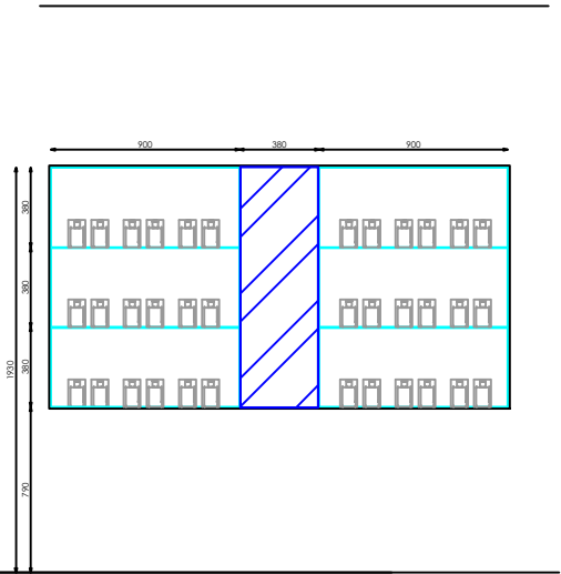
ALZADO FRONTAL
