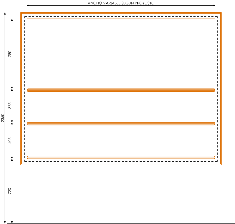
ALZADO
