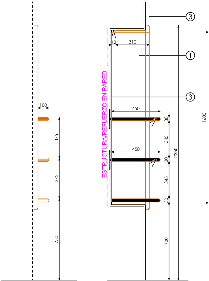
ALZADO LATERAL
