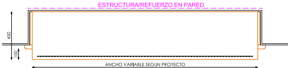
PLANTA SECCIONADA
