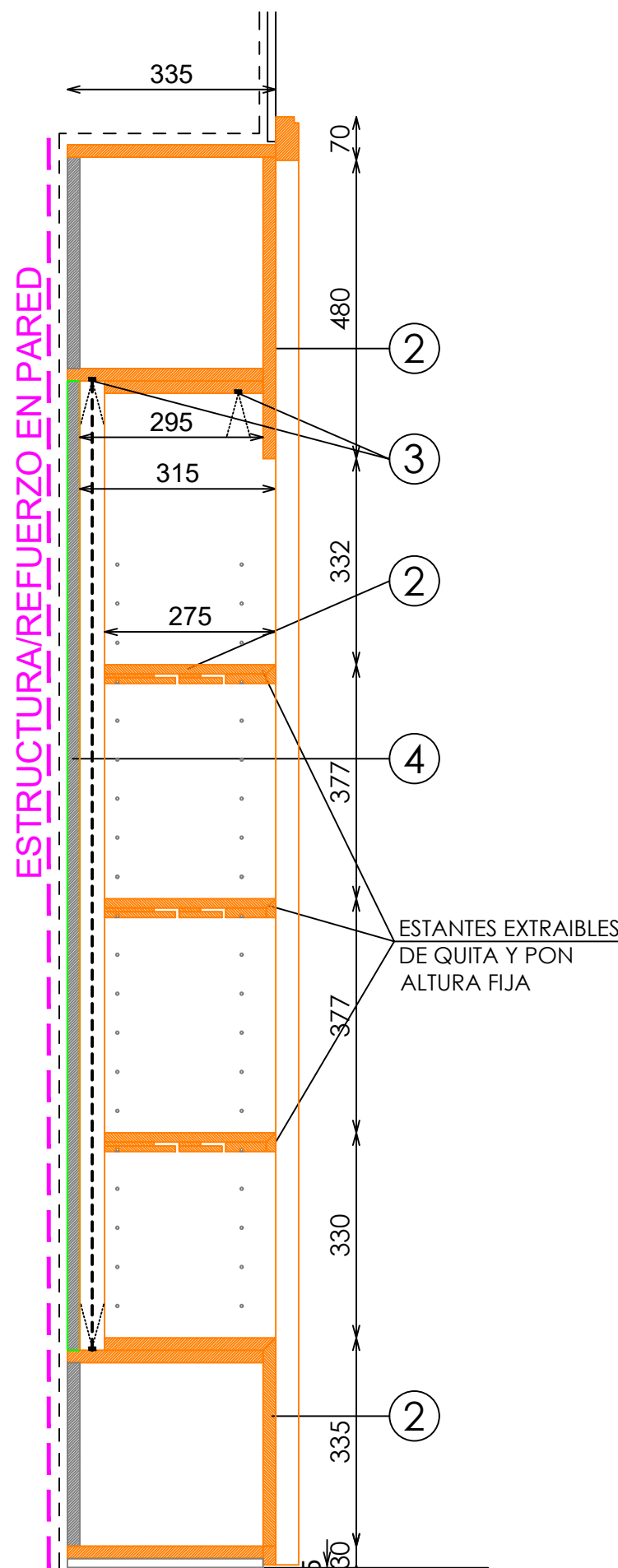
SECCIÓN (BALDAS)
