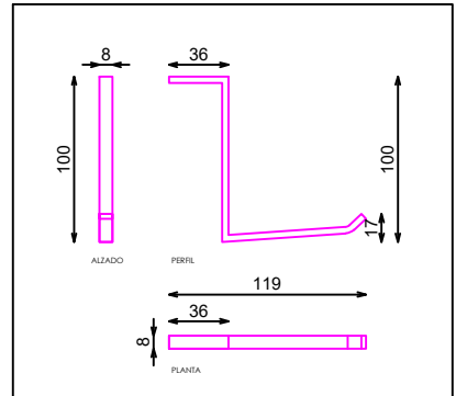
DET. PINCHO
