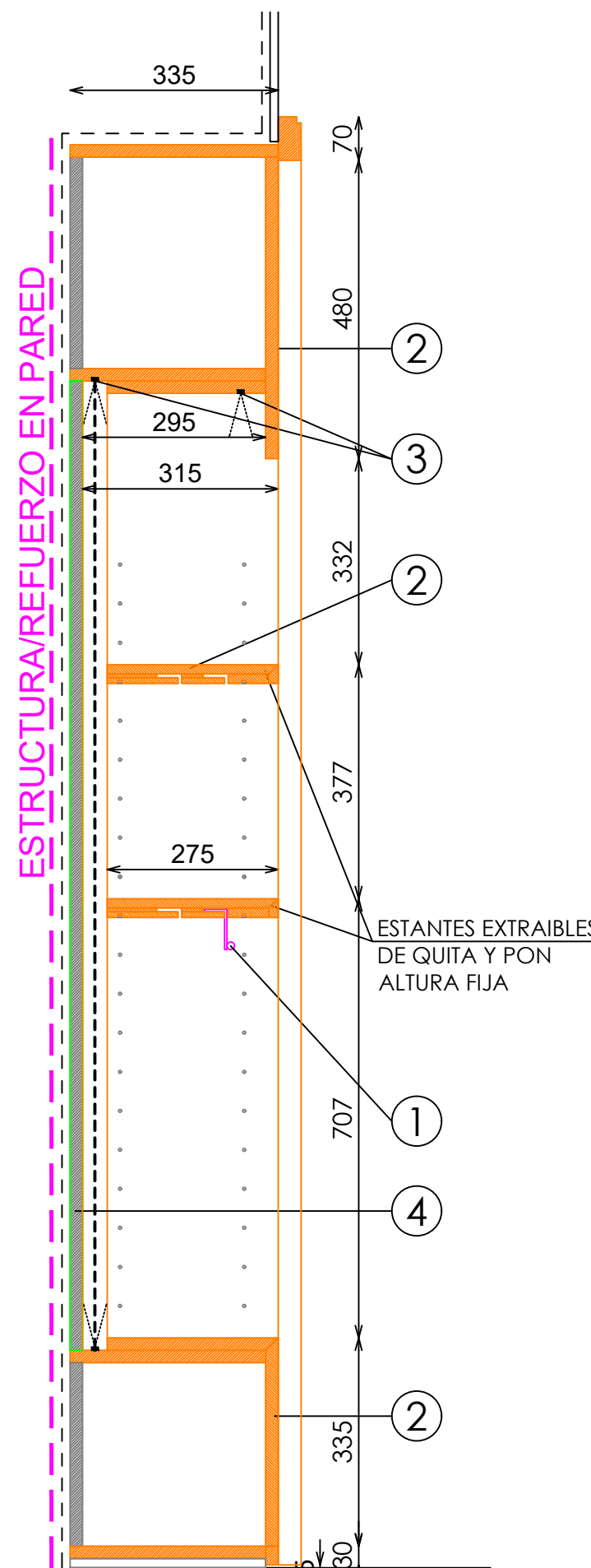
SECCIÓN (BARRA BOLSOS)
