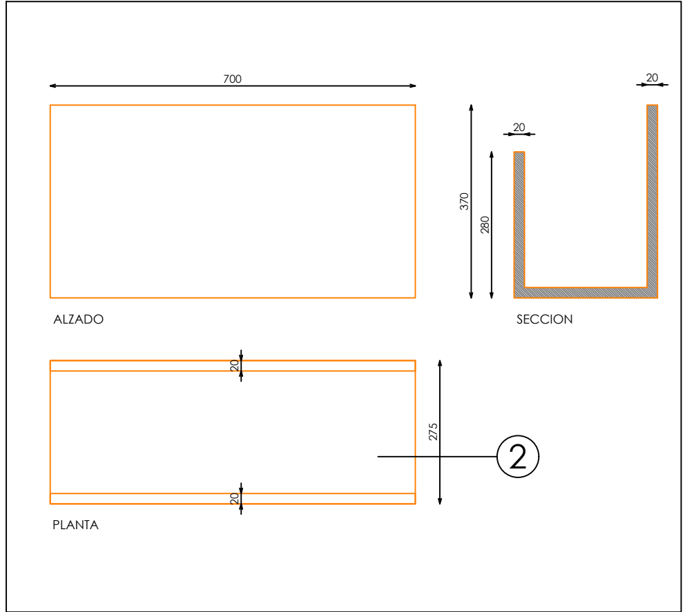
DET. CUBETA CINTURONES
