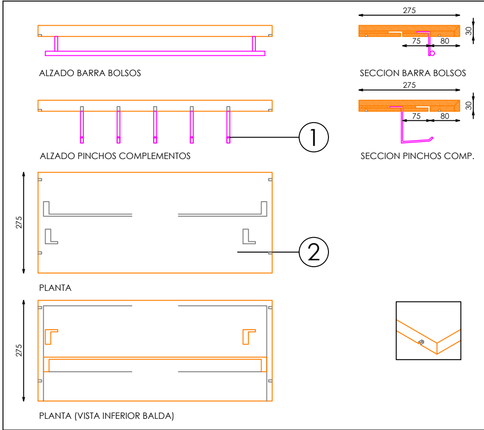
DET. BALDA EXTRAIBLE
