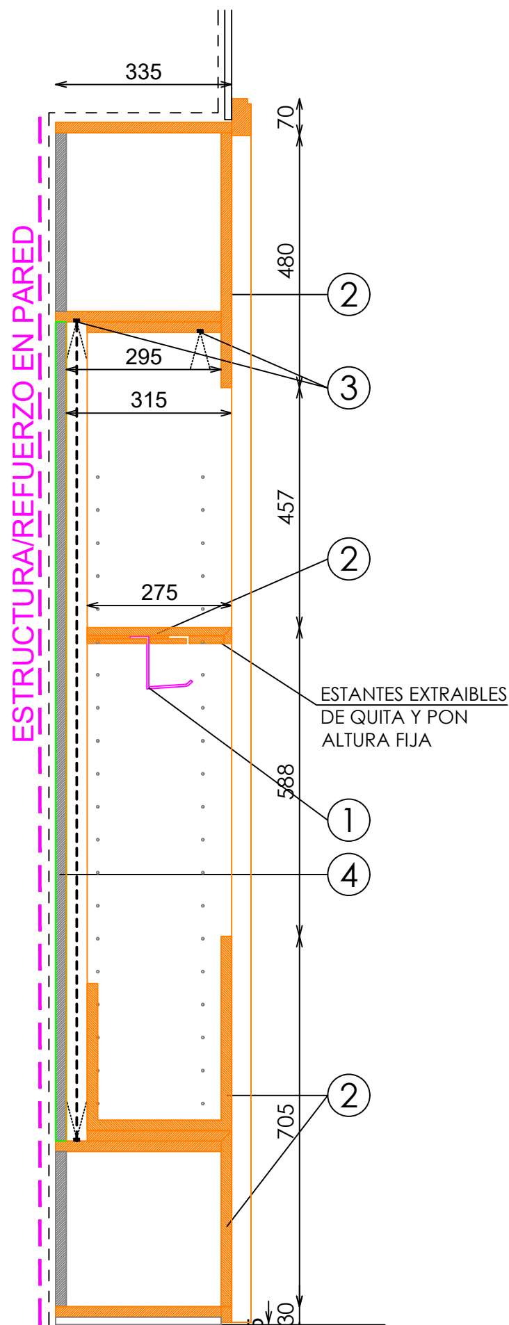
SECCIÓN (CINTURONES)
