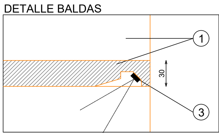
DETALLE BALDAS
