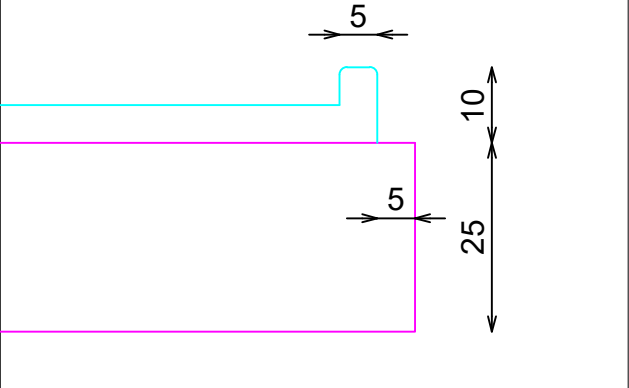
DETALLE SISTEMA ANCLAJE
