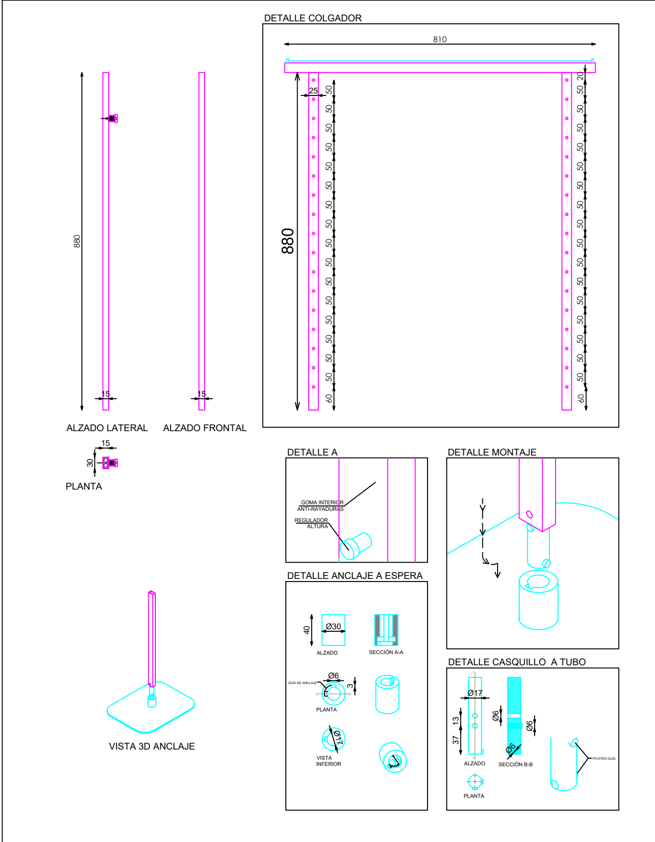
DETALLE COLGADOR INFERIOR EXTRAIBLE
