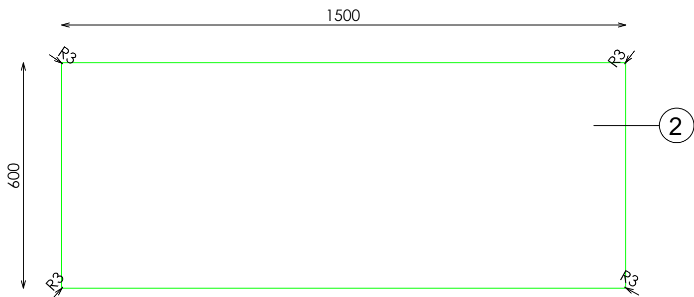
PLANTA
