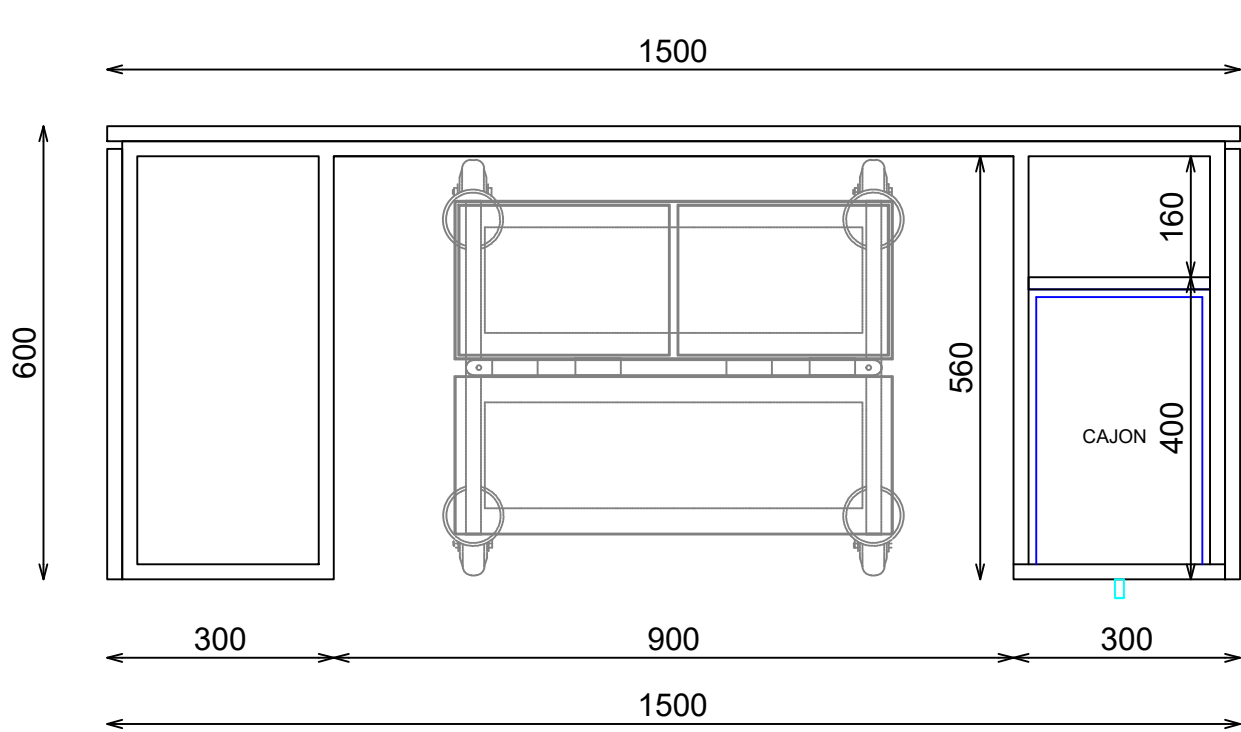
PLANTA SECCIONADA
