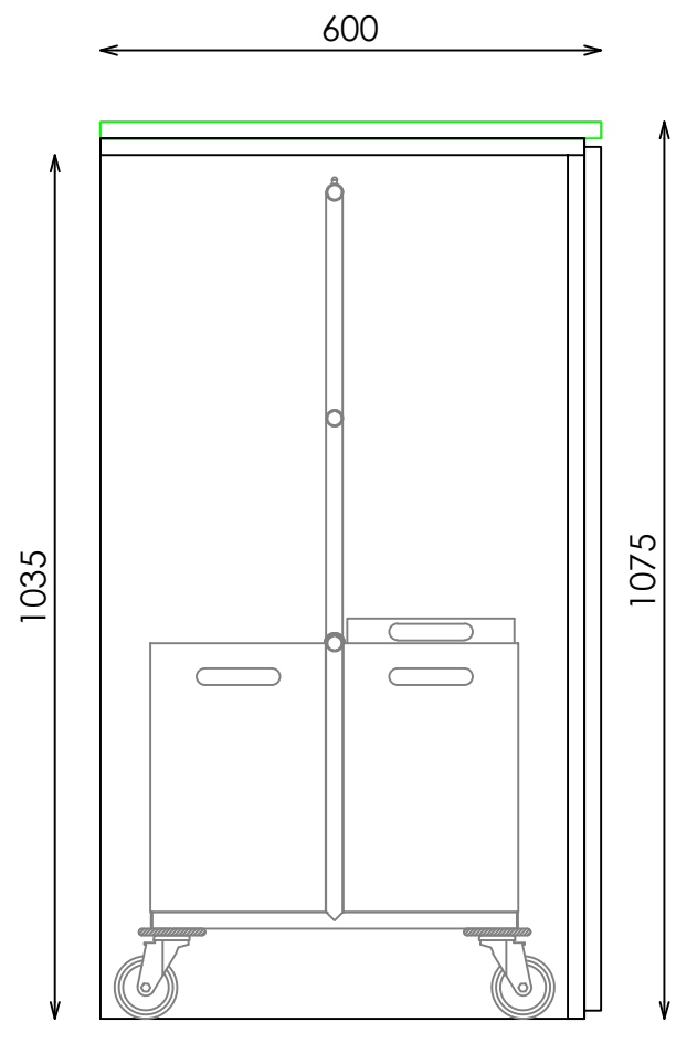
SECCION
