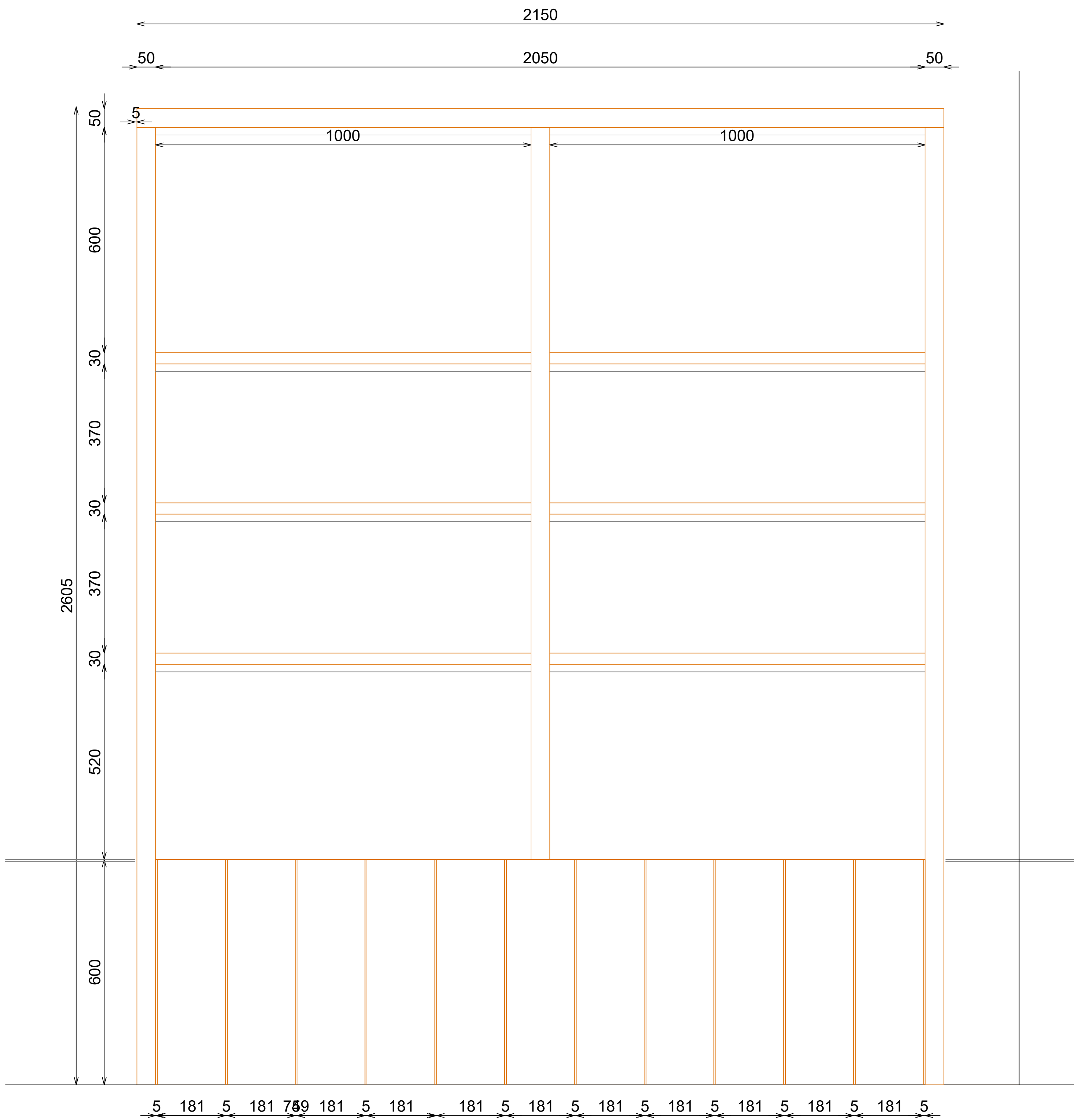
ALZADO
