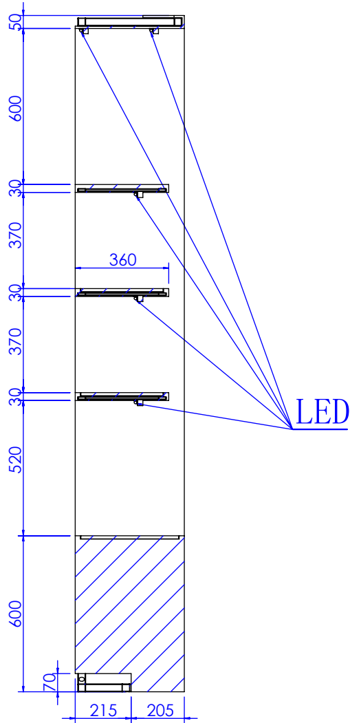
剖面 AG-AG
