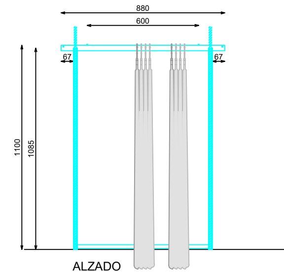
ALZADO
