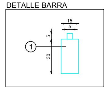
DETALLE BARRA
