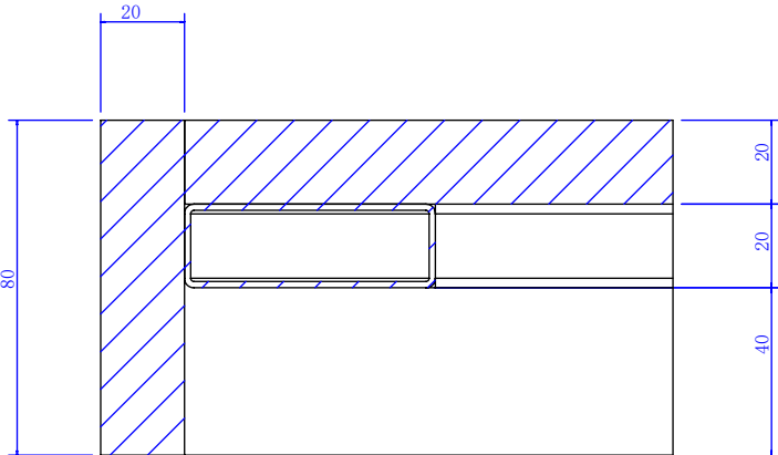
局部视图 B 比例 1 : 2
