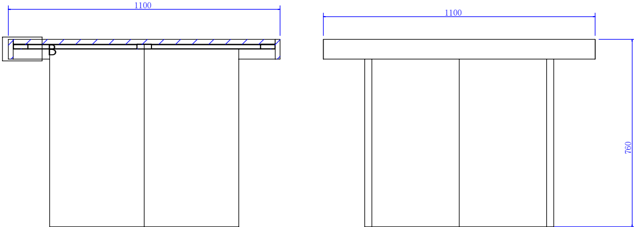
剖面 A-A
