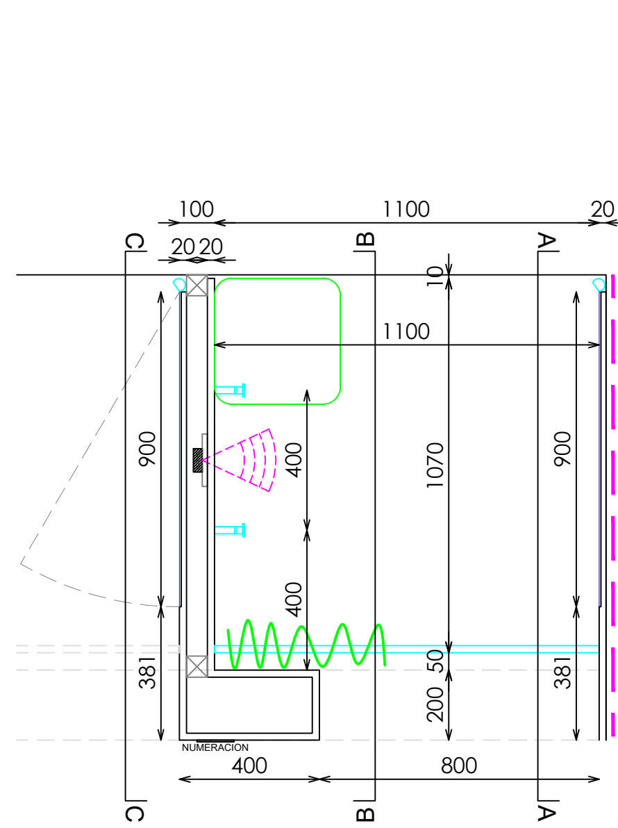
PLANTA
