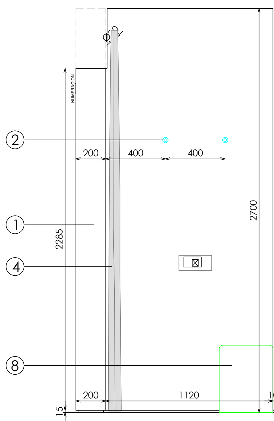
ALZADO LATERAL CUELGA (B-B)
