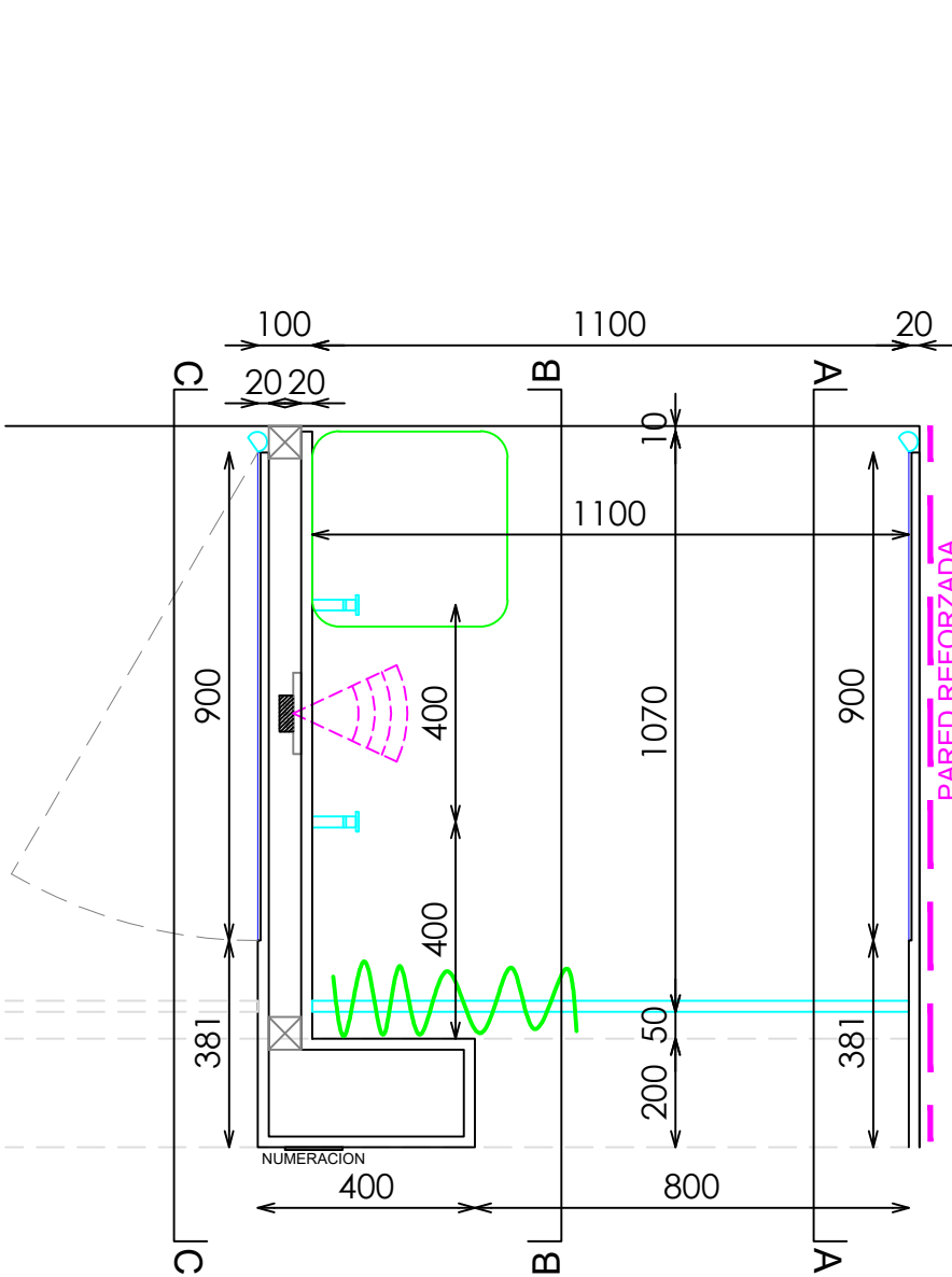
PLANTA
