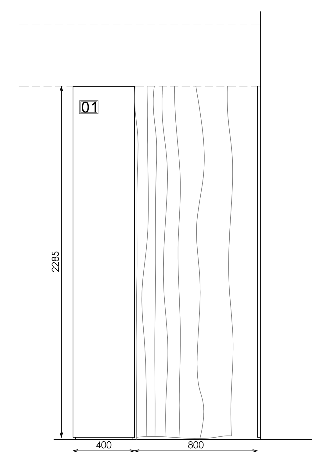
ALZADO
