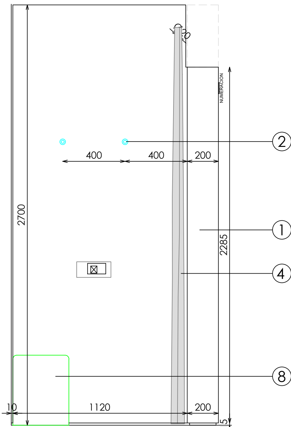
ALZADO LATERAL CUELGA (B-B)
