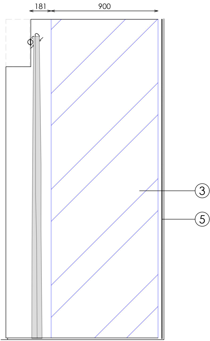
ALZADO LATERAL ESPEJO (A-A)
