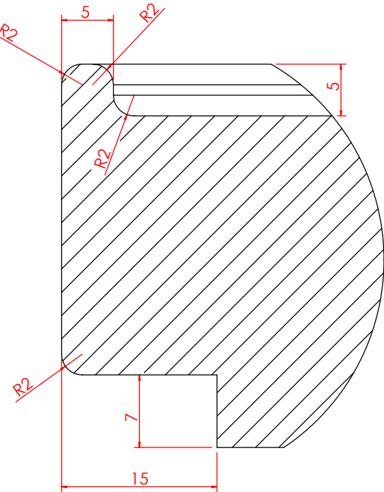
局部视图 AH 比例 2 : 1
