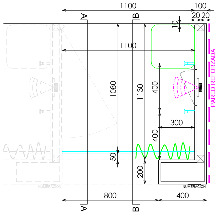
PLANTA
