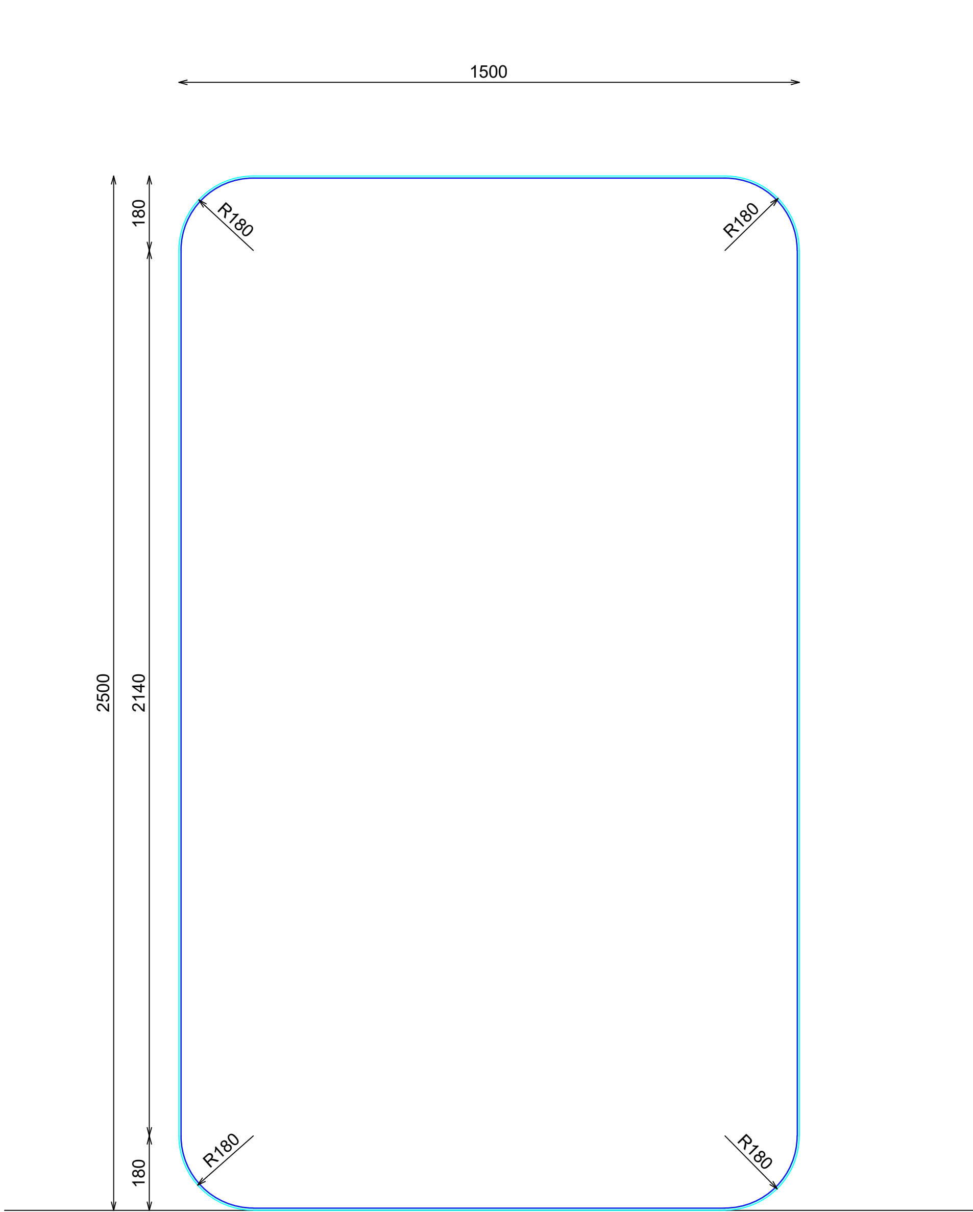
ALZADO
