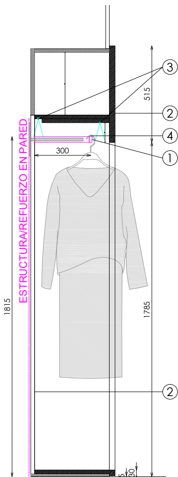
SECCIÓN BARRA ALTA
