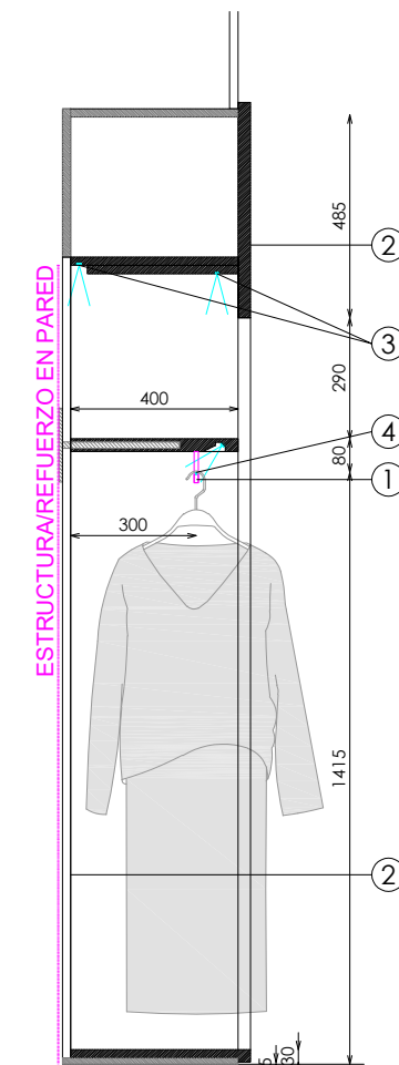
SECCIÓN BARRA BAJA + ESTANTE
