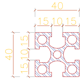
5 节点 1:2 DETAIL
