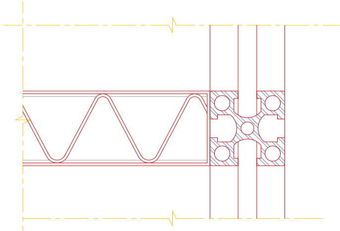
7 节点 1:2 DETAIL
