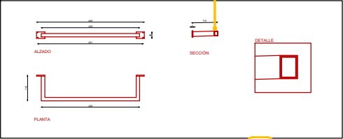
DETALLE BARRA 220 (MODULO 45)
