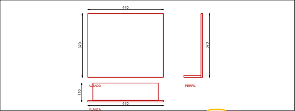
DETALLE BARRA 110 (MODULO 45)
