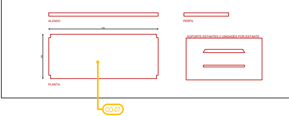
DETALLE ESTANTE (MODULO 65)
