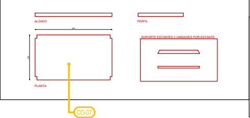
DETALLE ESTANTE (MODULO 45)
