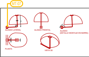
DETALLE BARRA 110 (MODULO 65)
