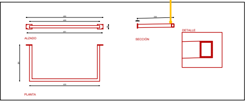
DETALLE BARRA 220 (MODULO 45)
