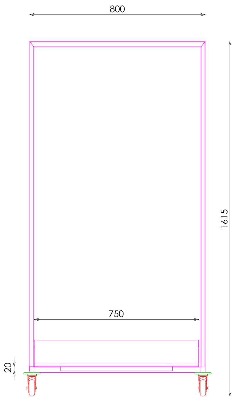
ALZADO FRONTAL
