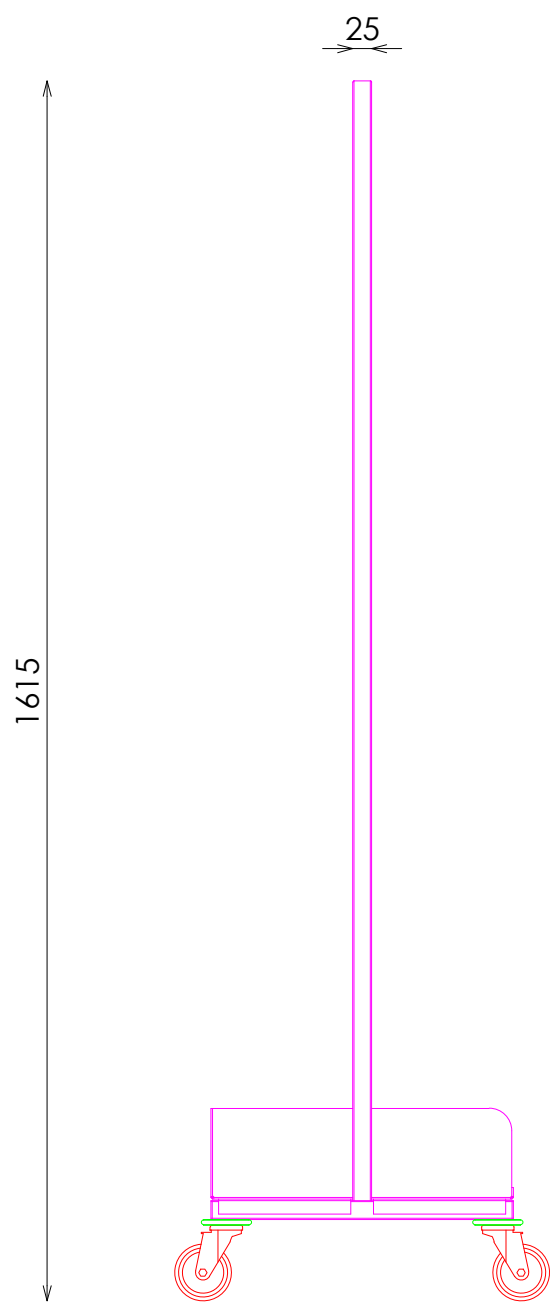
ALZADO LATERAL
