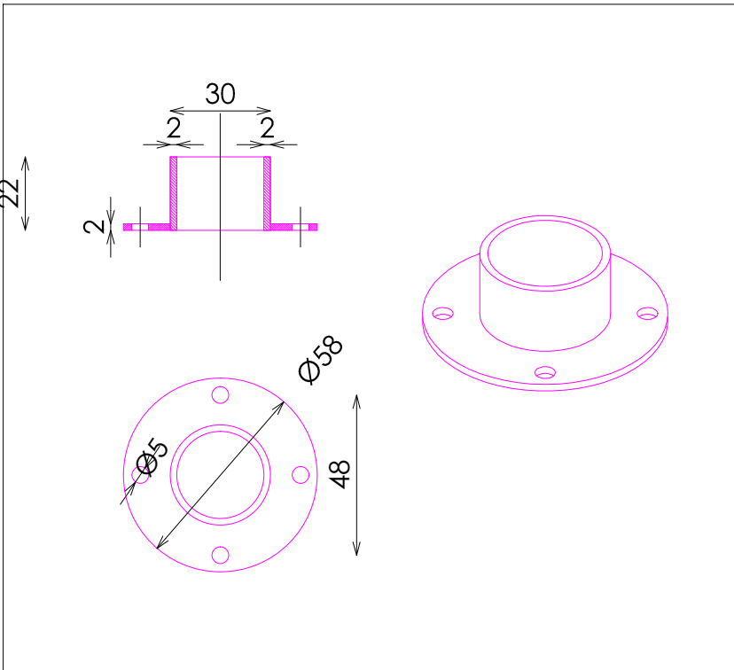
CASQUILLO EMBELLECEDOR
