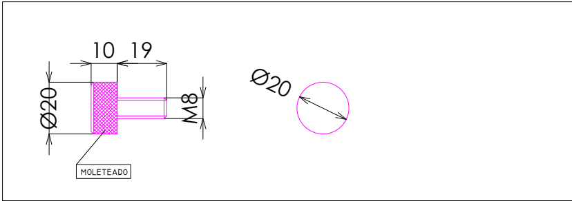
TONILLO MOLETEADO
