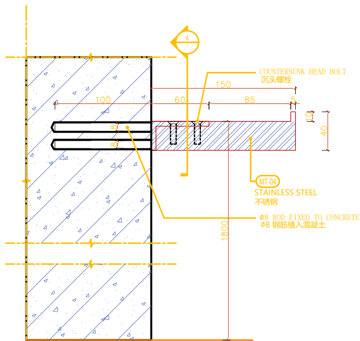
2 支撑杆件放大正立面 1:2 BAR HOLDER ENLARGE FRONT ELEVATION
