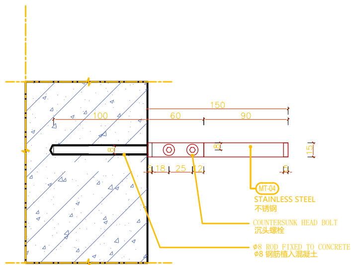
1 支撑杆件放大平面 1:2 BAR HOLDER ENLARGE PLAN
