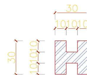
5 节点 1:2 DETAIL
