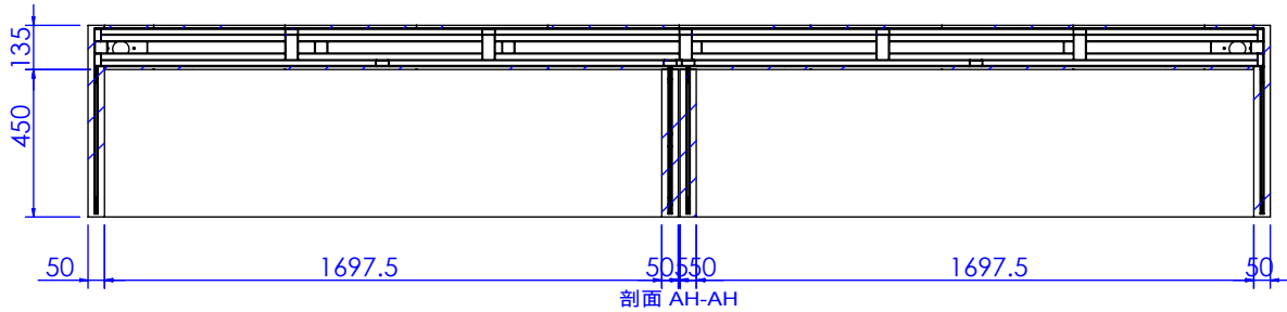
剖面 AH-AH
