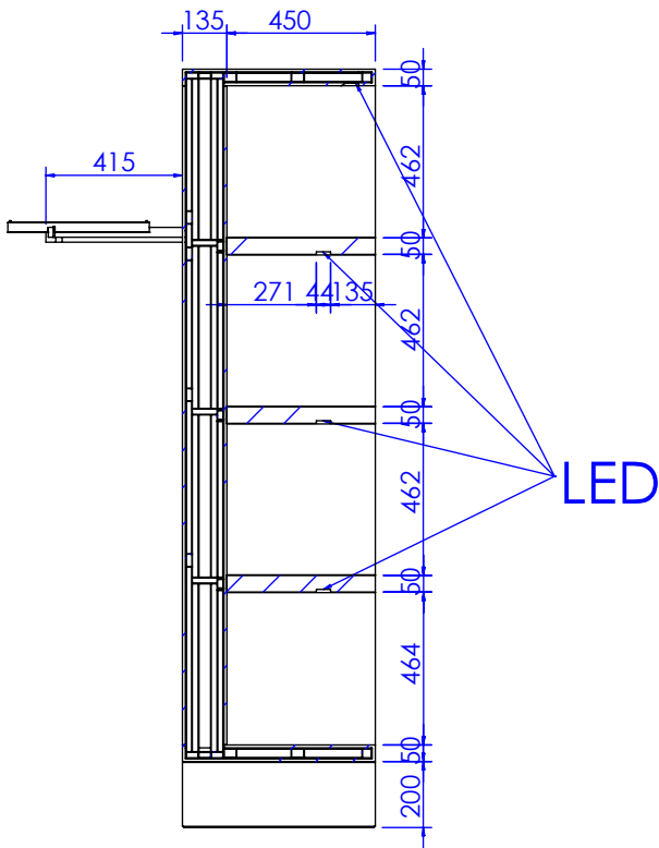
剖面 AG-AG
