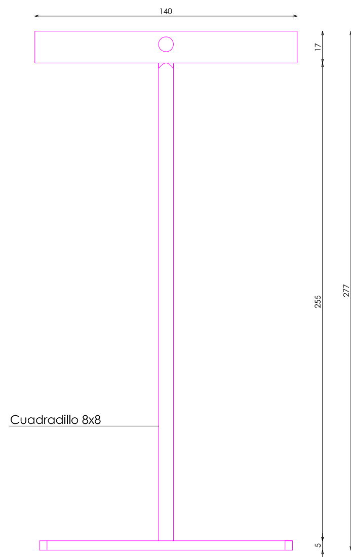
ALZADO
