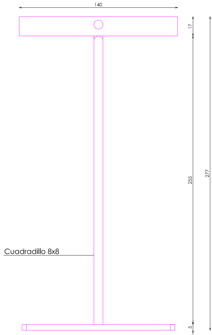
ALZADO
