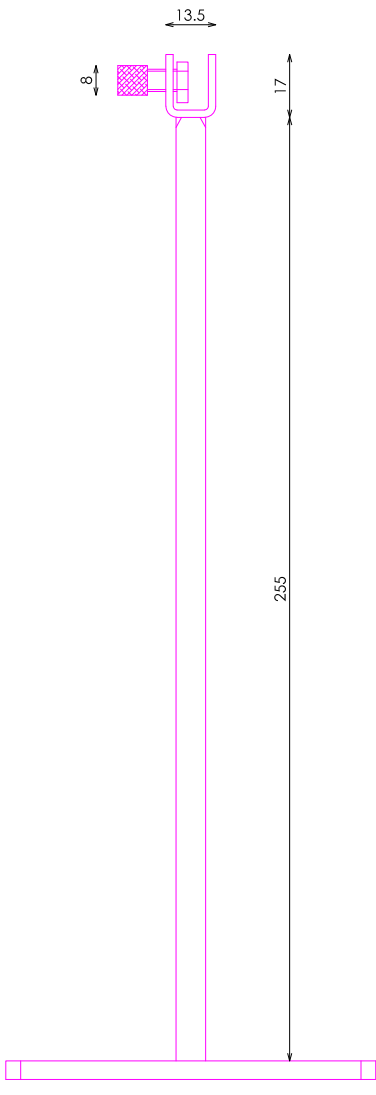
PERFIL
