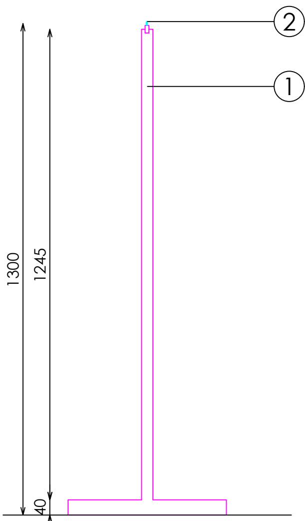
SECCIÓN
