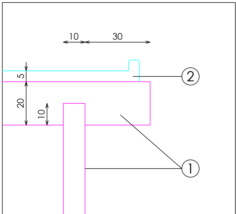
DETALLE B
