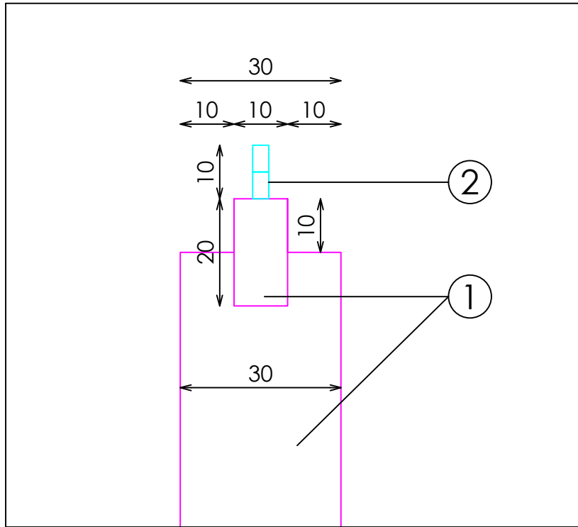
DETALLE A
