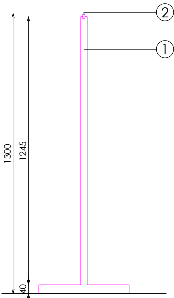
SECCIÓN
