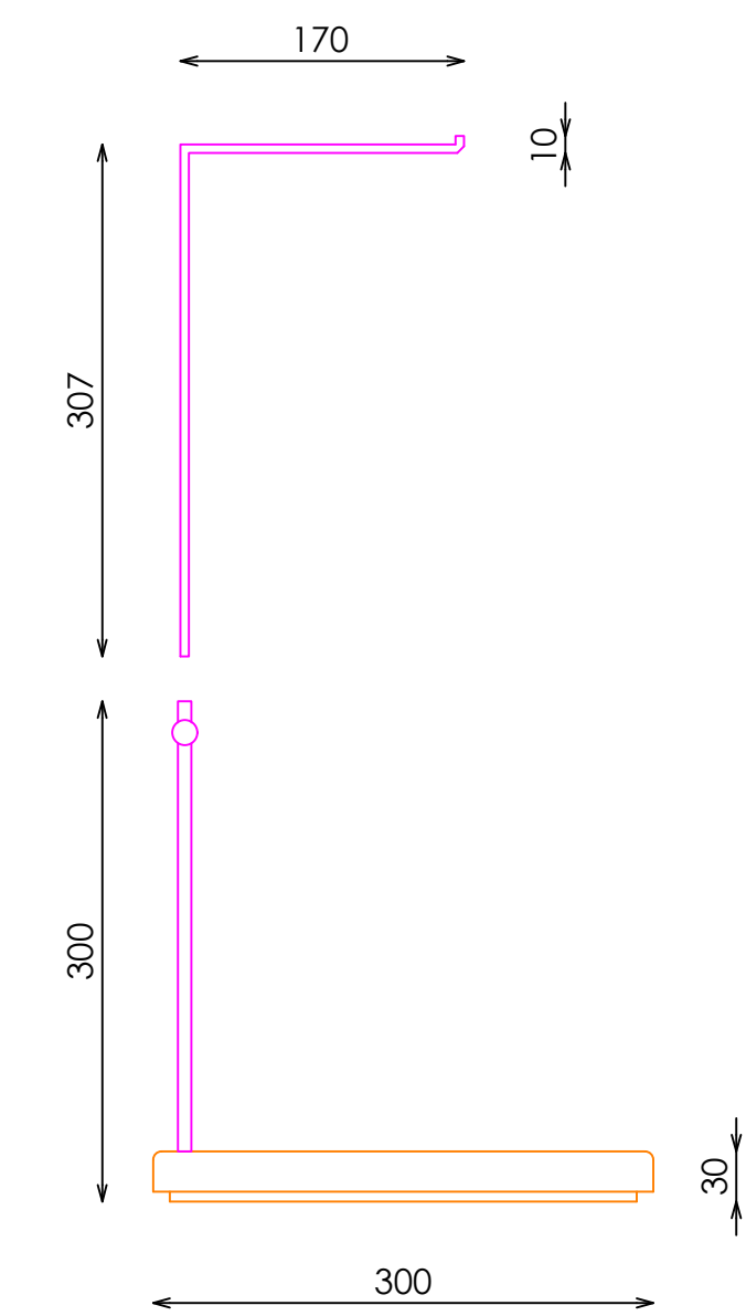
ALZADO
