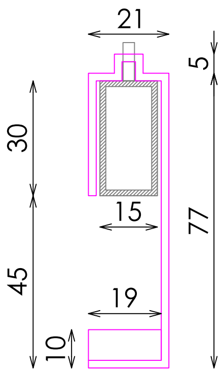
SECCIÓN
