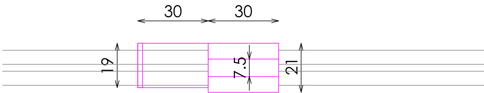
PLANTA
