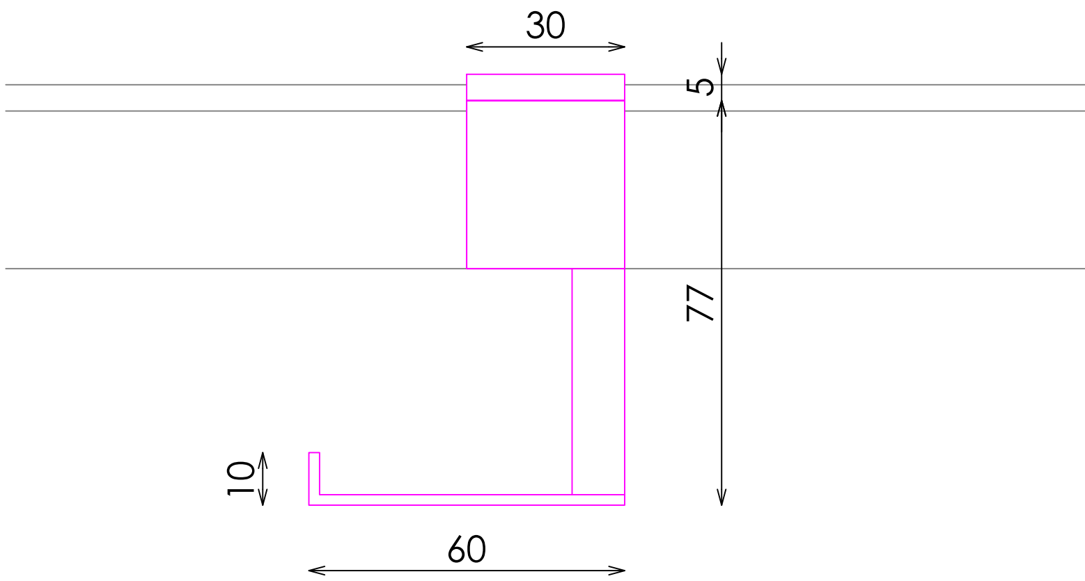
ALZADO
