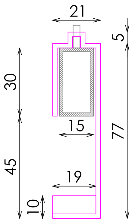
SECCIÓN
