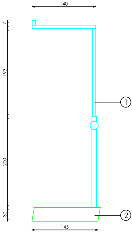
PERFIL
