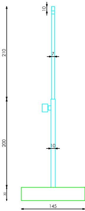
ALZADO
