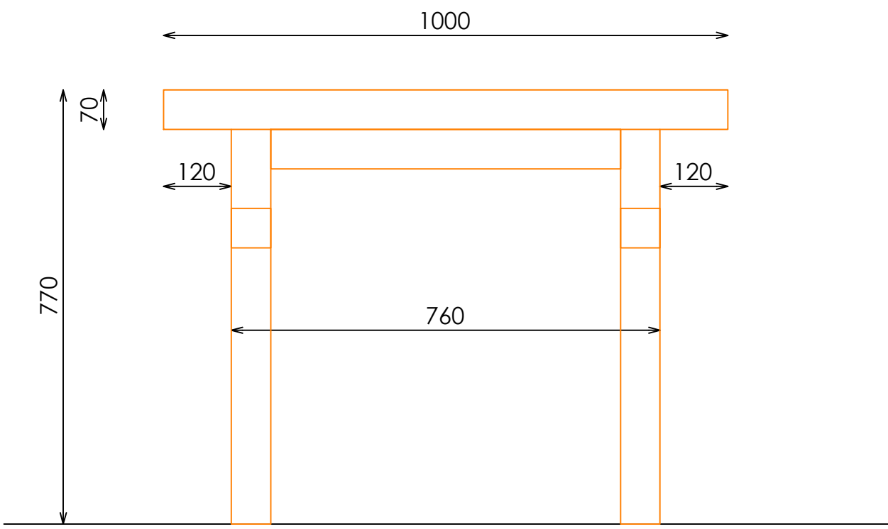
ALZADO LATERAL
