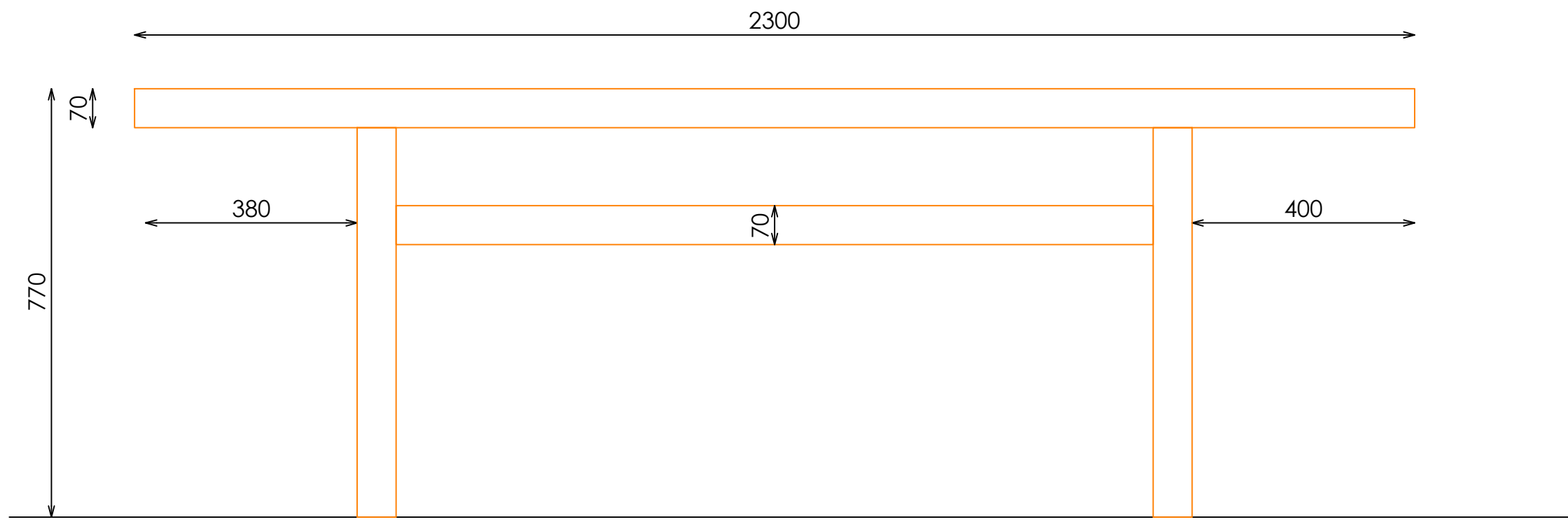
ALZADO FRONTAL
