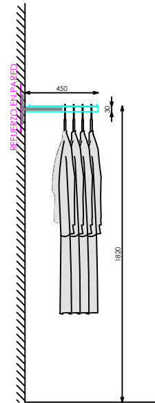
SECCION
