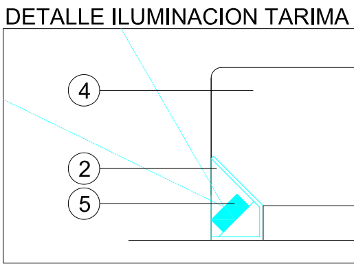
DETALLE ILUMINACION TARIMA
