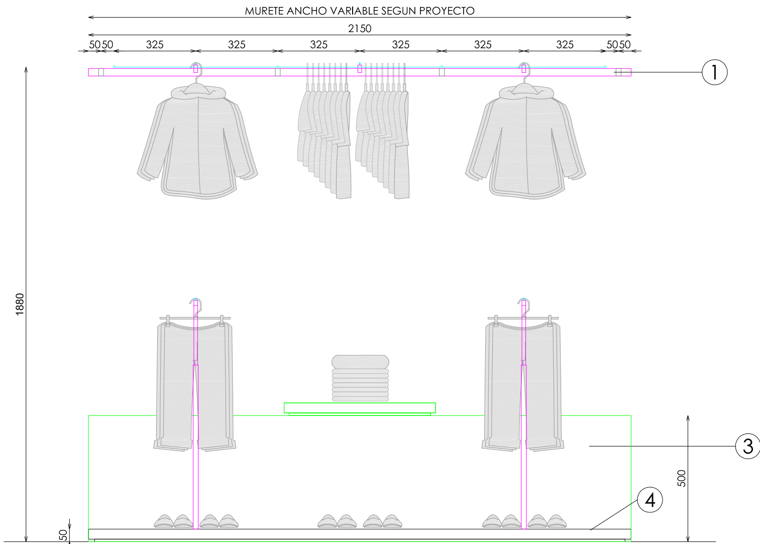
ALZADO FRONTAL
