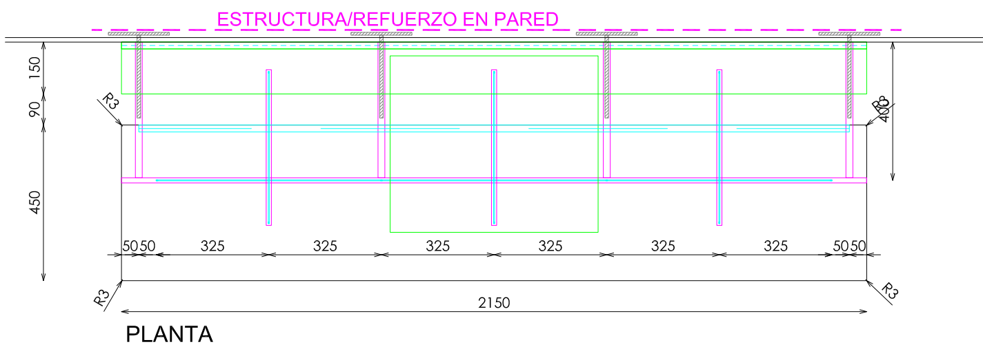
PLANTA
