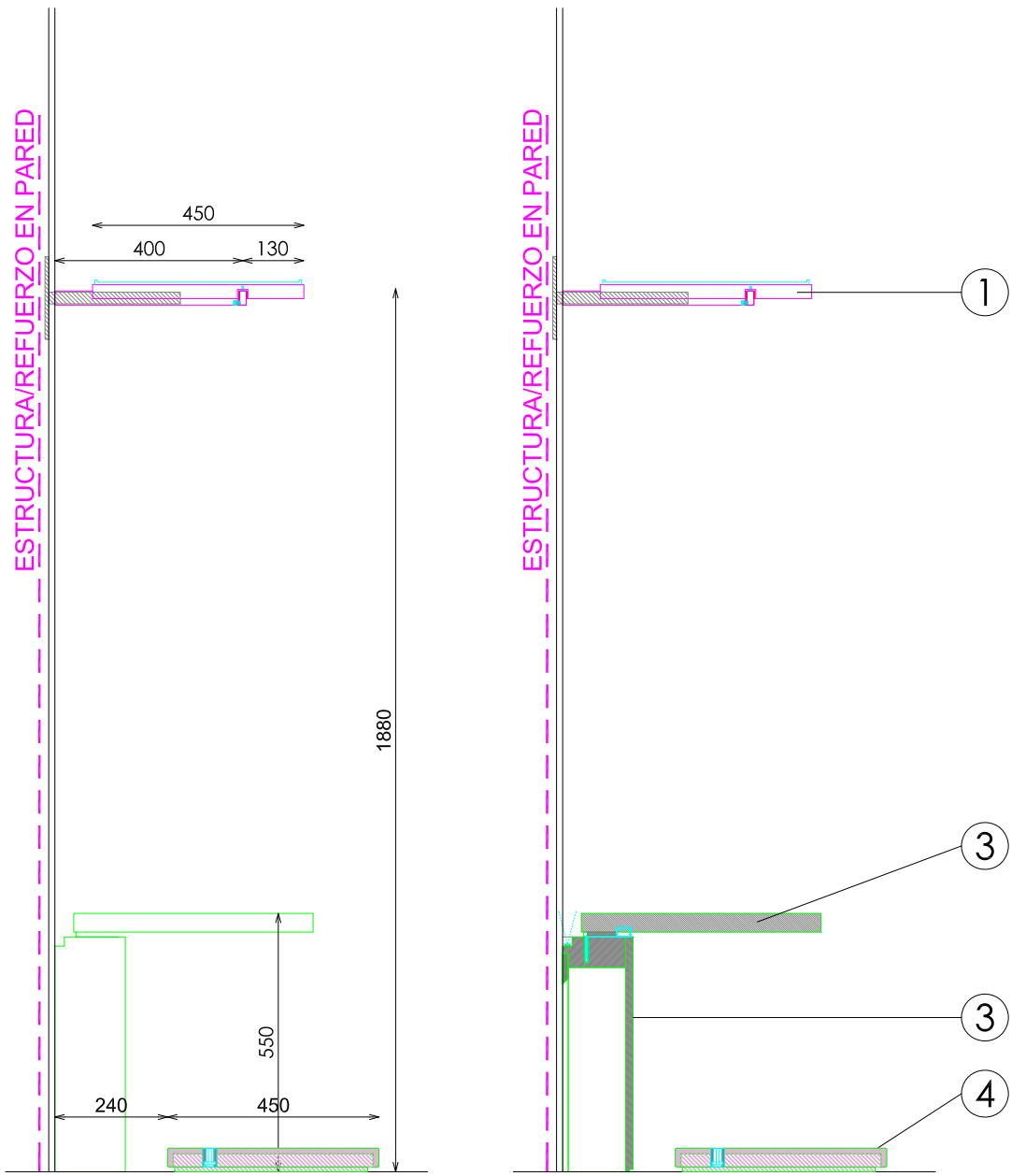
PERFIL
