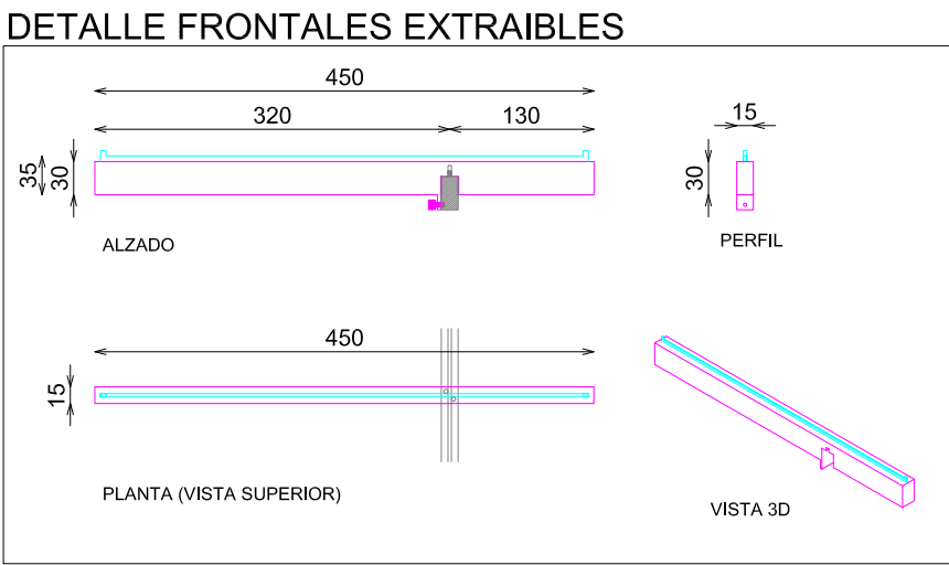
DETALLE FRONTALES EXTRAIBLES
