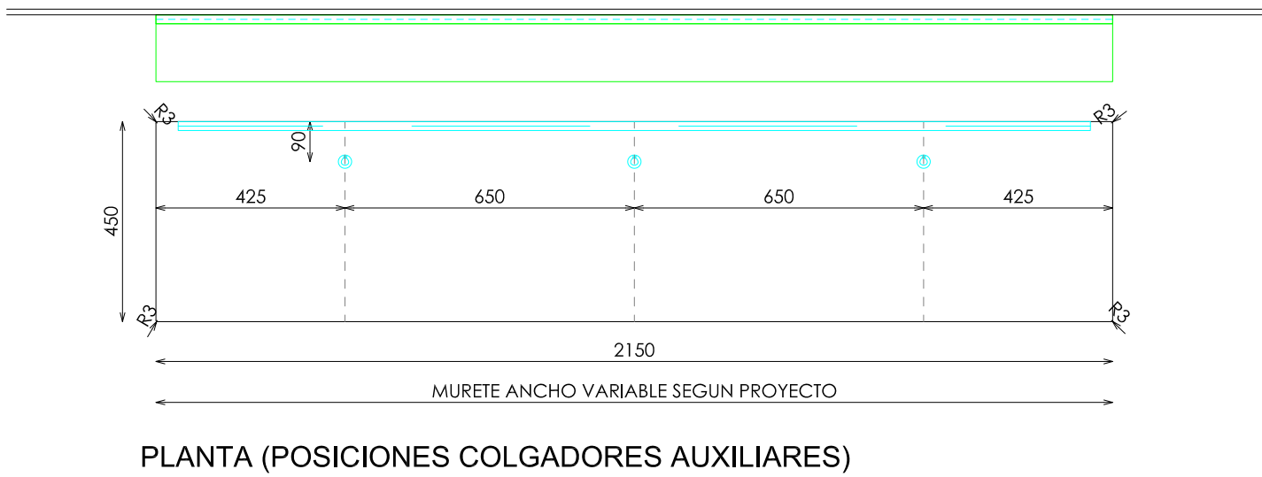
PLANTA (POSICIONES COLGADORES AUXILIARES)
