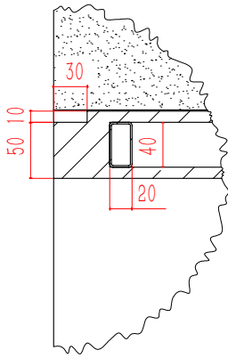
局部视图 C
